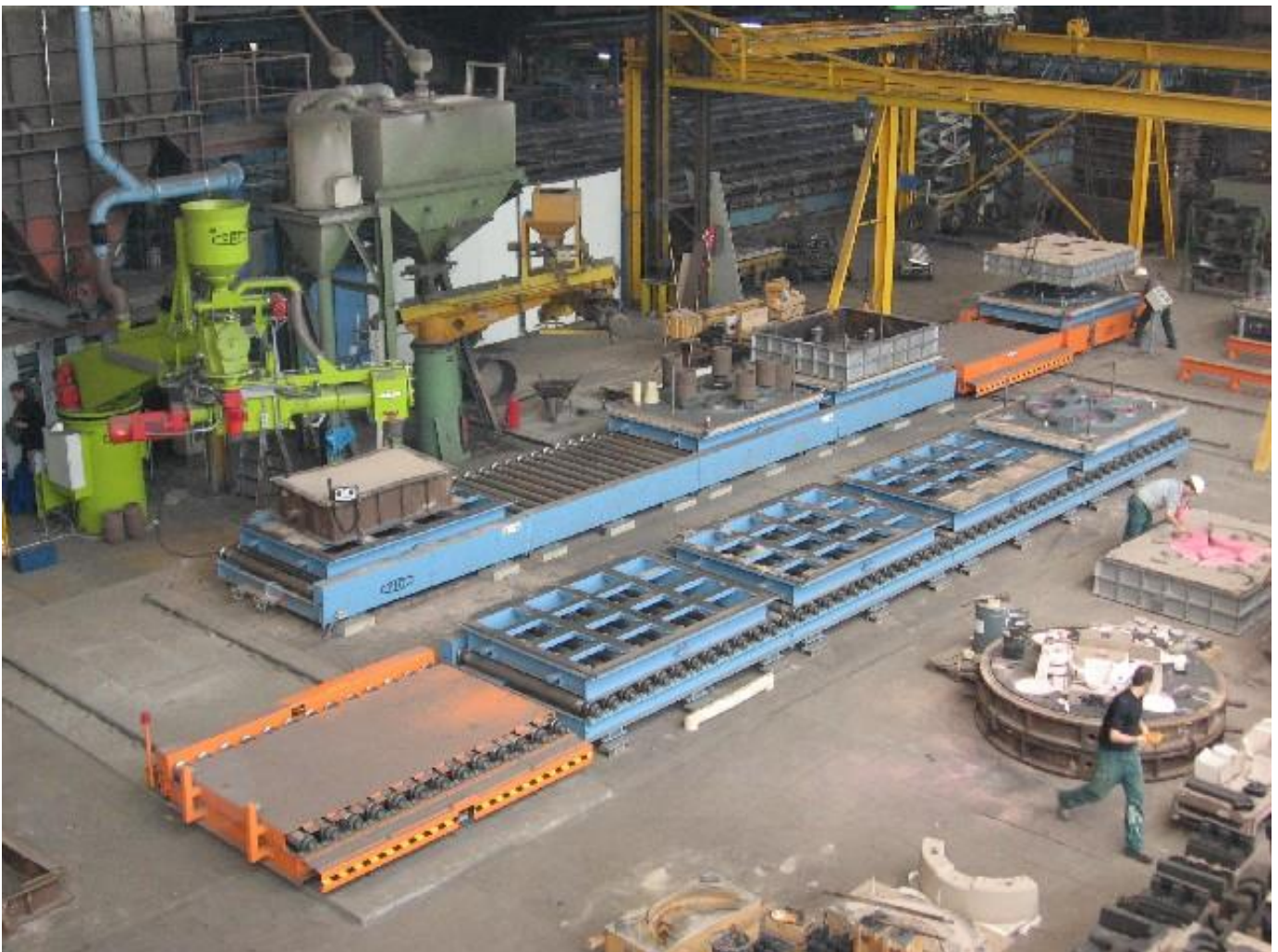
Bild 7: teil-automatisierte Kaltharz-Formanlage (FWH, Mülheim)
